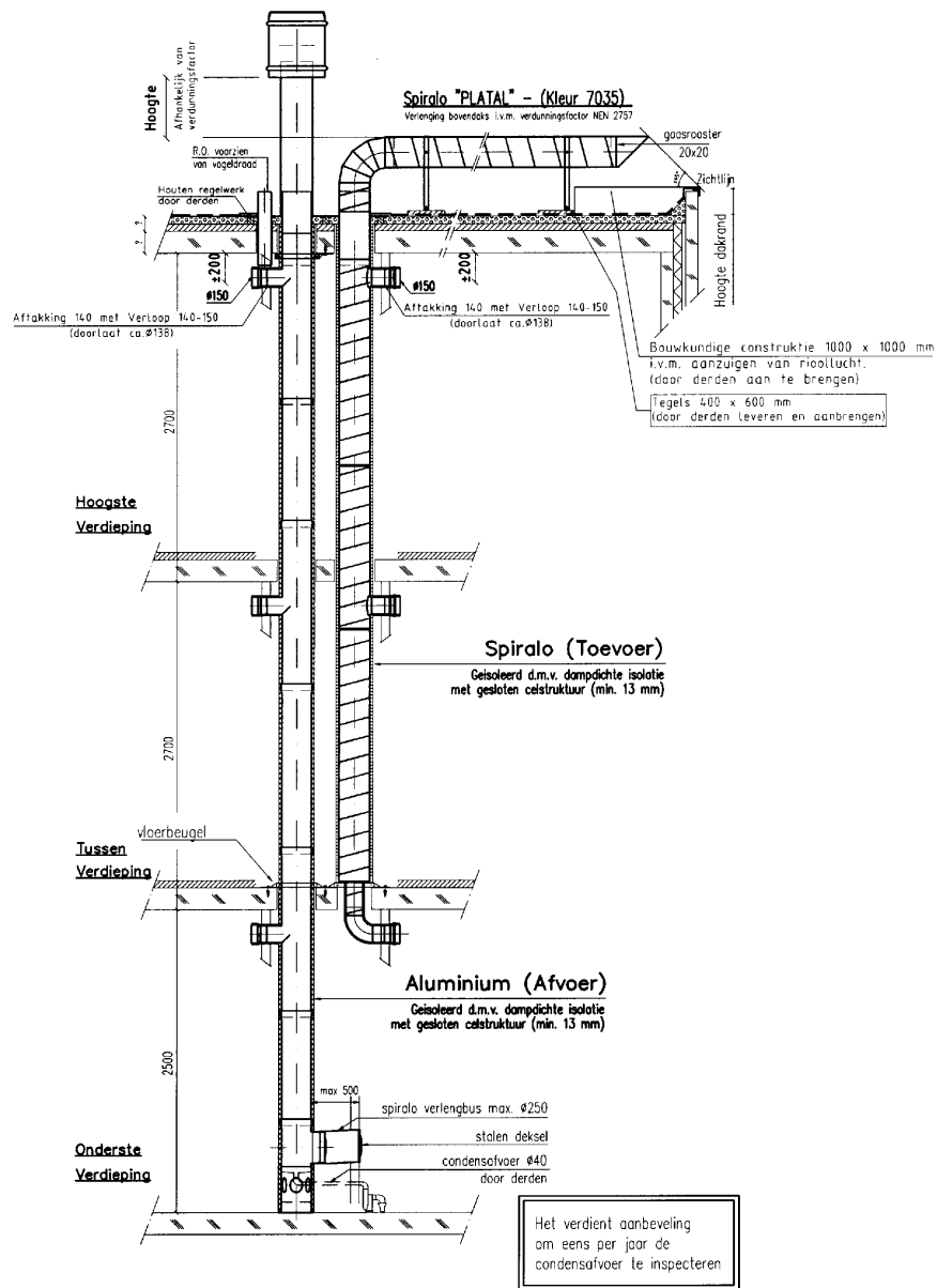
WTW-systeem met LT-kanaal voor de dakrand
